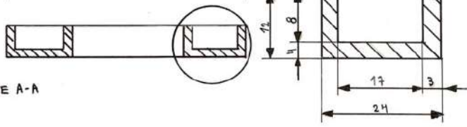
DETALLE Esc 1:1
